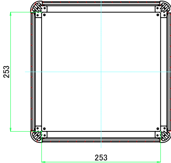
C-C ( 1 : 5 )
