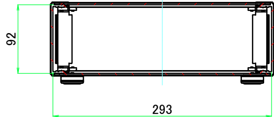
A-A ( 1 : 5 )
