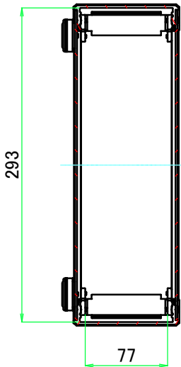
B-B ( 1 : 5 )
